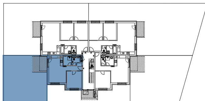
PÔDORYS PODLAŽIA
